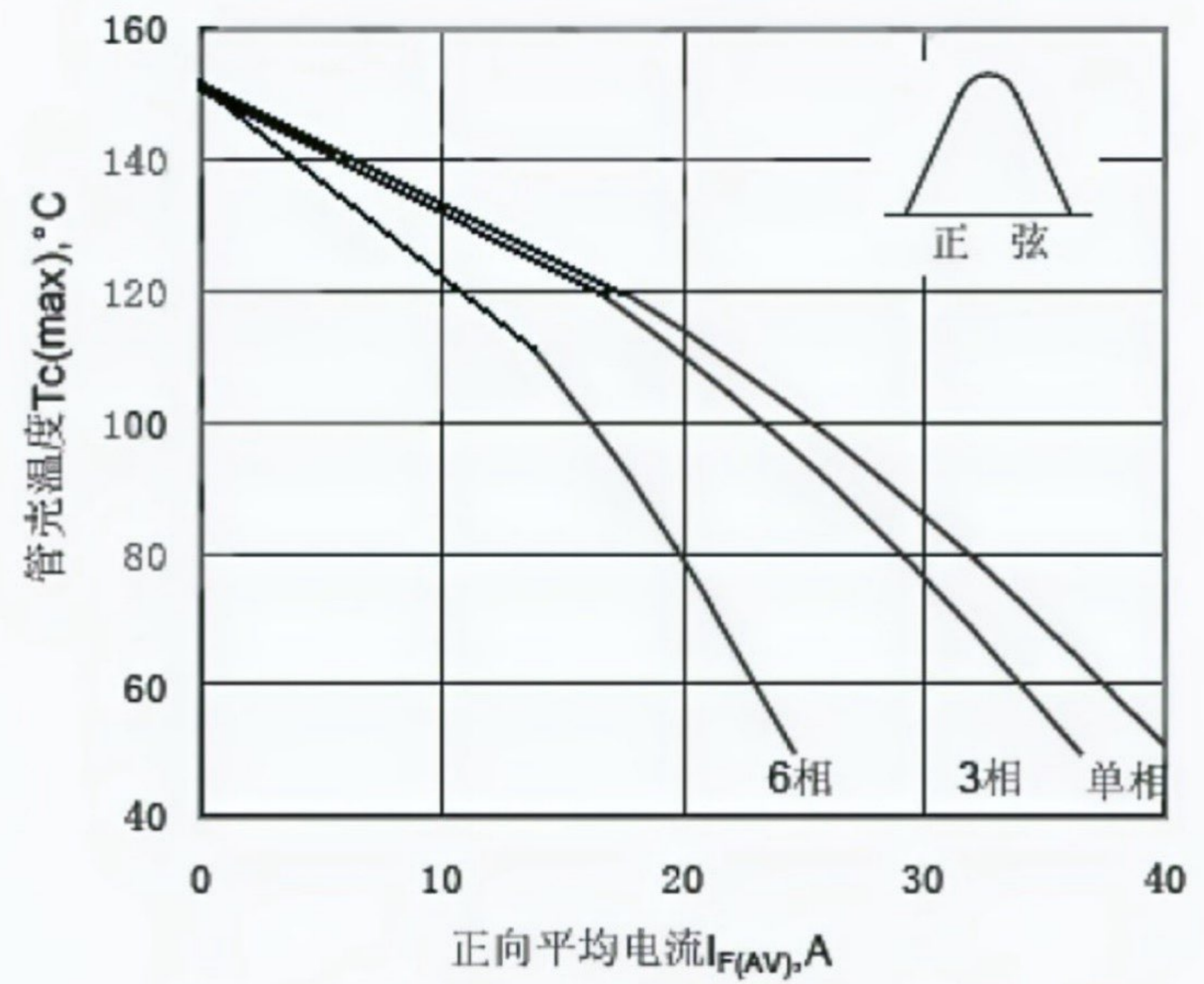
Fig.4 管壳温度与正向平均电流关系曲线
