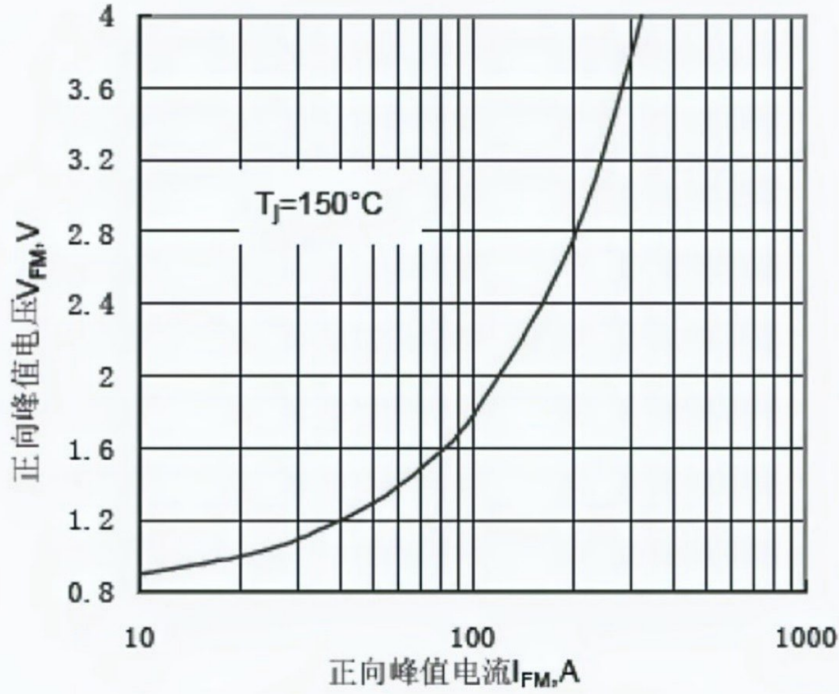
Fig.1 正向伏安特性曲线
