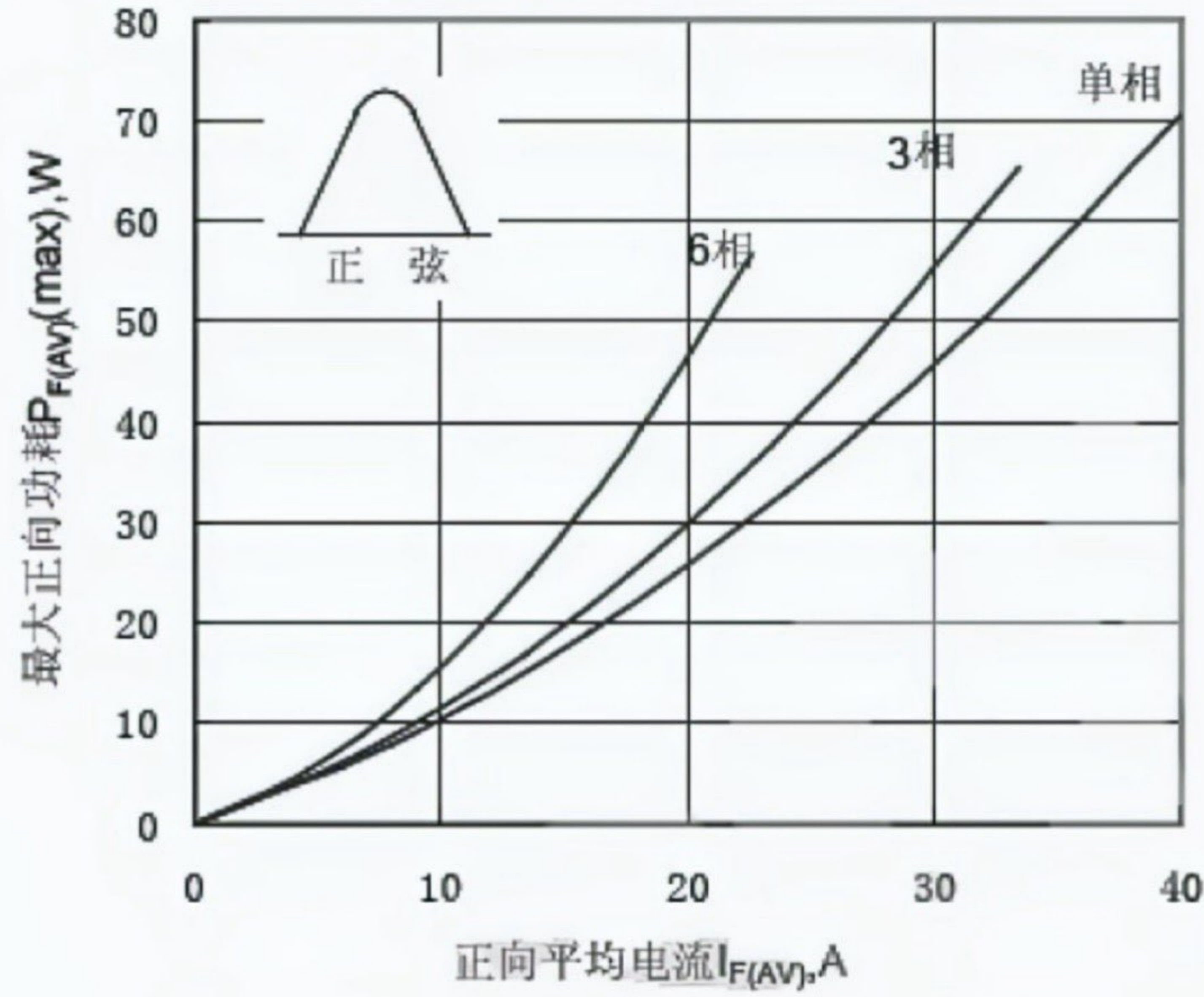
Fig.3 最大正向功耗与平均电流关系曲线
