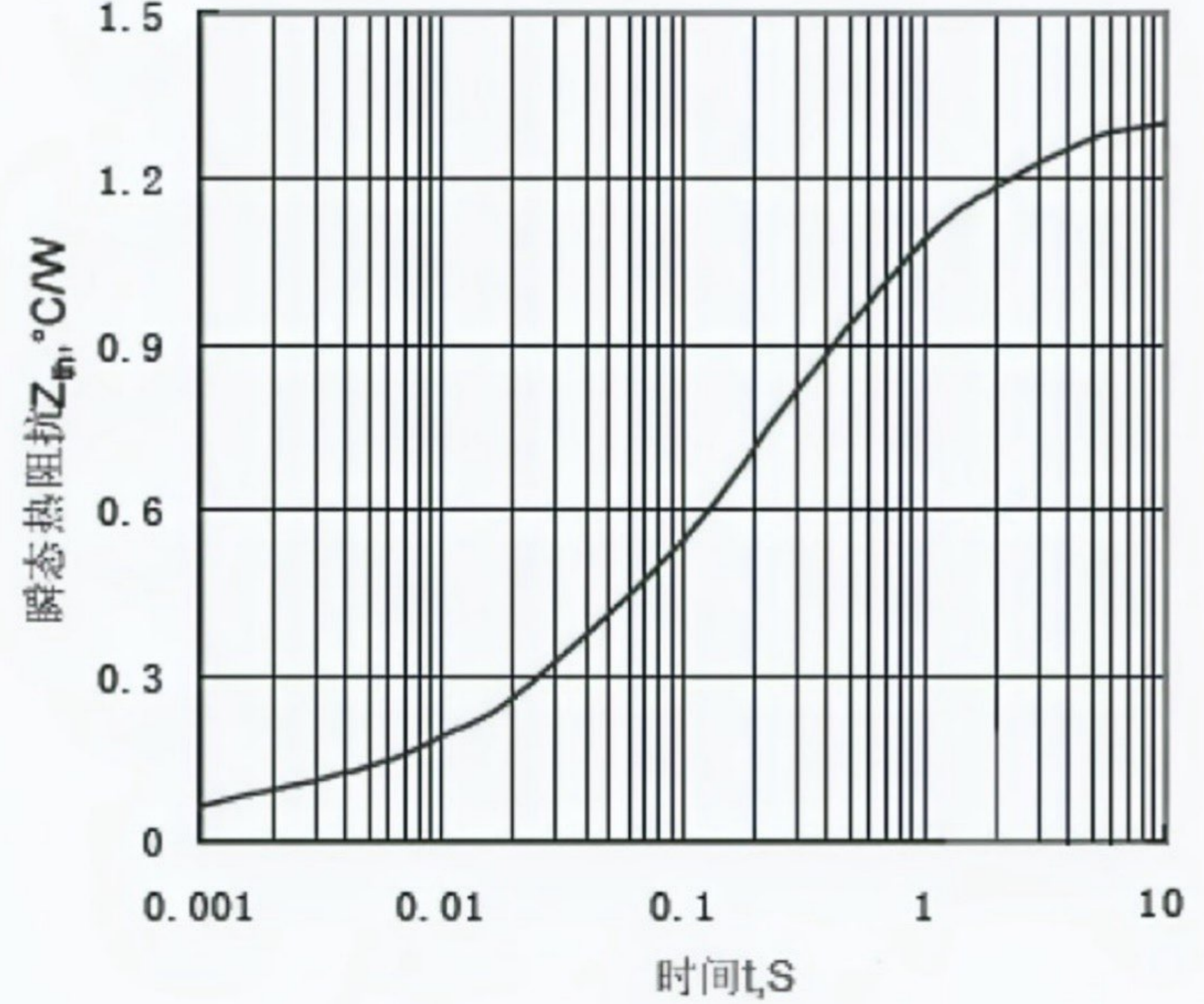
Fig.2 瞬态热阻抗曲线
