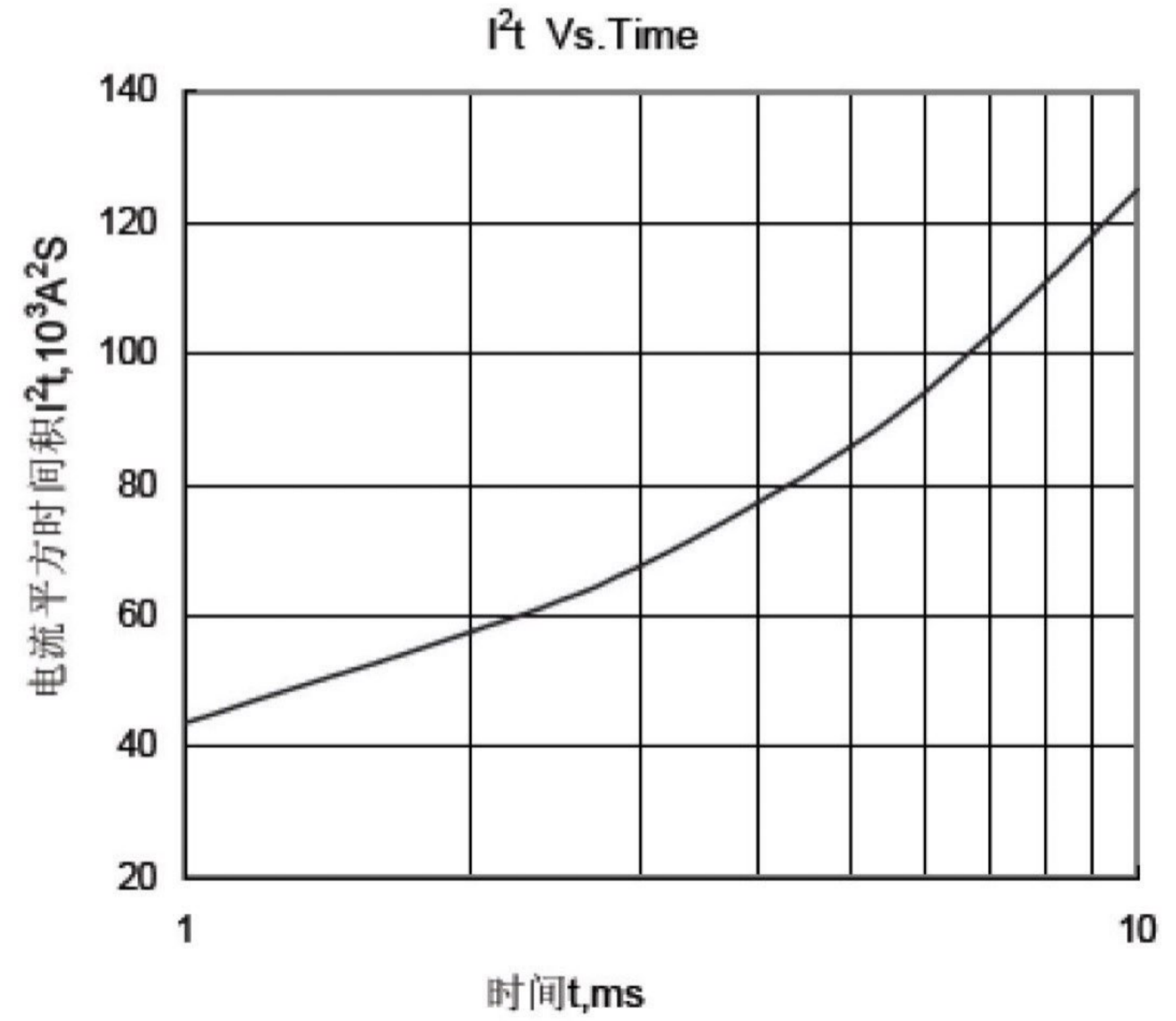
Fig.8 I^2t 特性曲线
