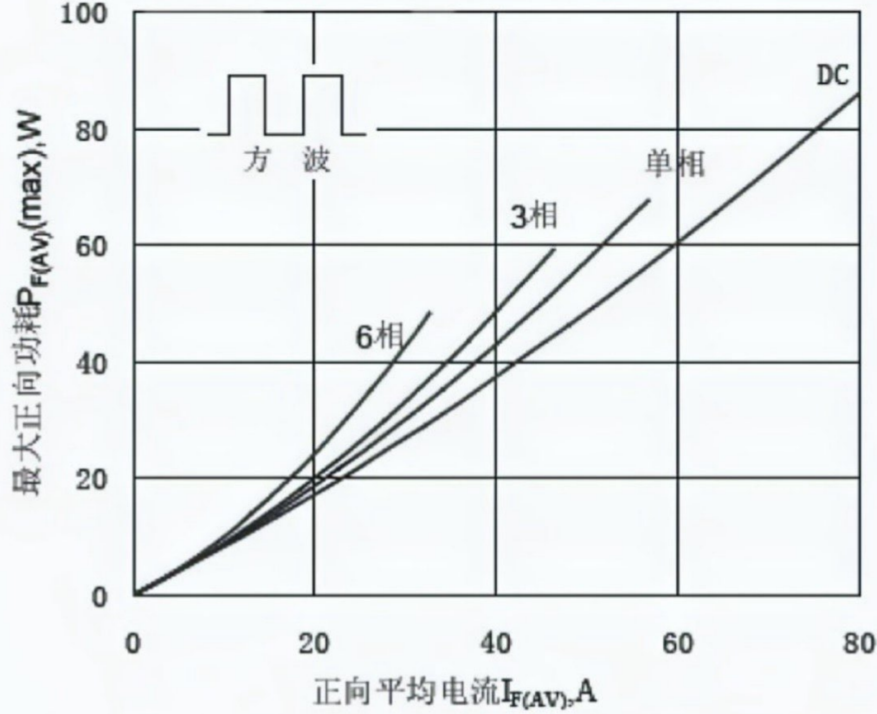
Fig.5 最大正向功耗与平均电流关系曲线
