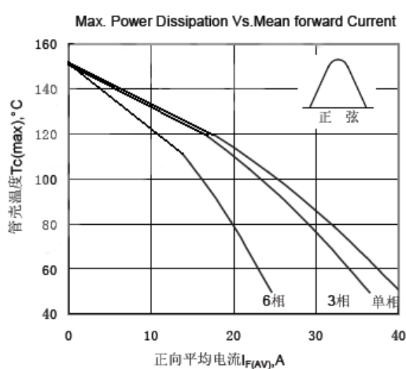
Fig.4 管壳温度与正向平均电流关系曲线
