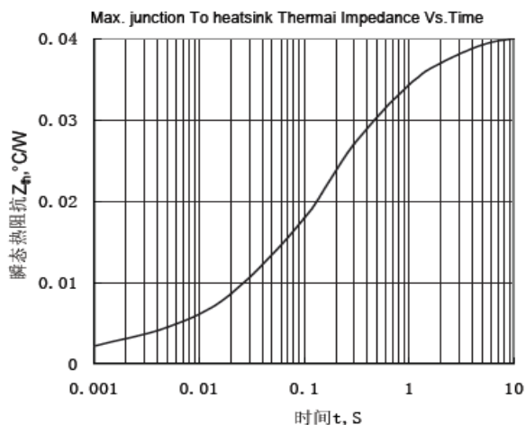
Fig.2 结至散热器瞬态热阻抗曲线
