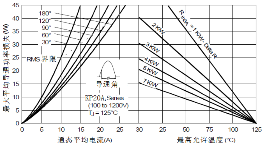
Fig. 3 - 通态损耗特性
