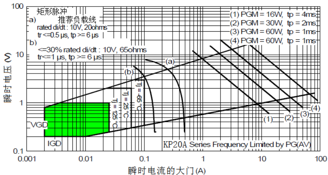
Fig. 16 - 栅极特性
