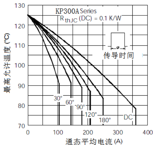
图 5 额定电流特性
