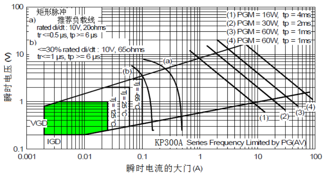
Fig. 16 - 栅极特性
