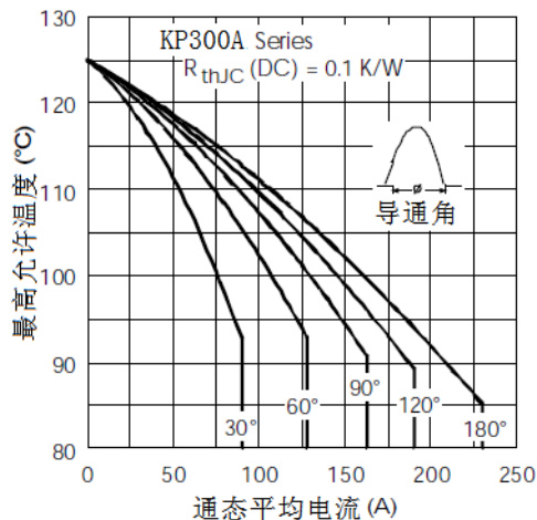
图 4 额定电流特性
