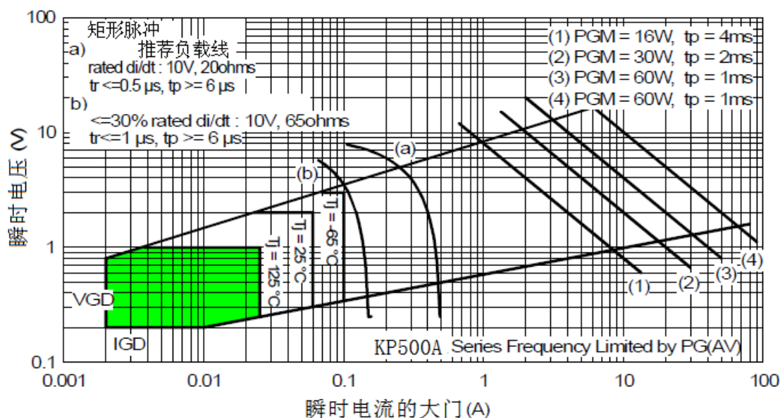
Fig. 16 - 栅极特性
