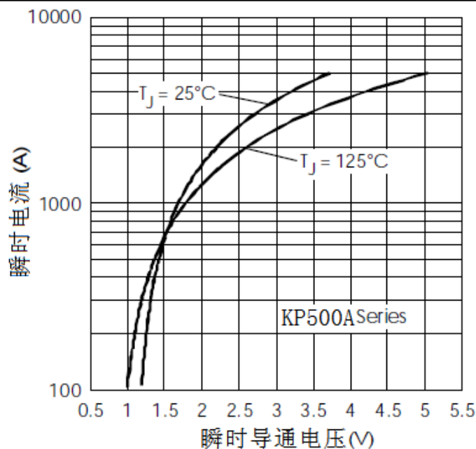
Fig. 7 - 正向压降特性
