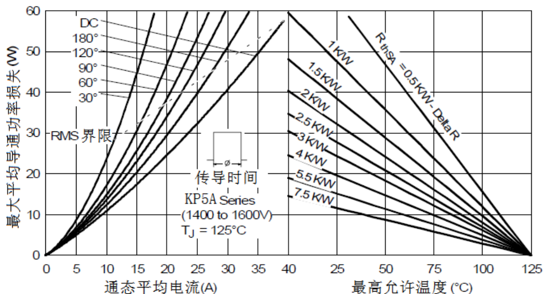
Fig. 11 - 通态损耗特性
