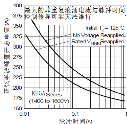
Fig. 13 - 最大反向浪涌电流
